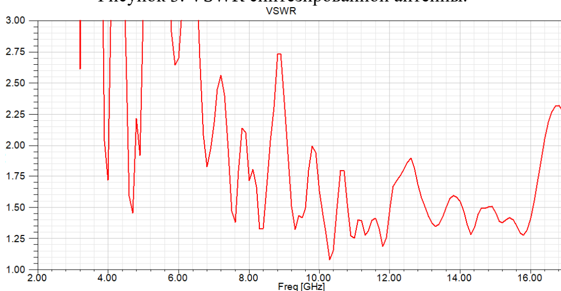
Рисунок 3. Фрагмент частотной зависимости VSWR в диапазоне 2-17 ГГц.
