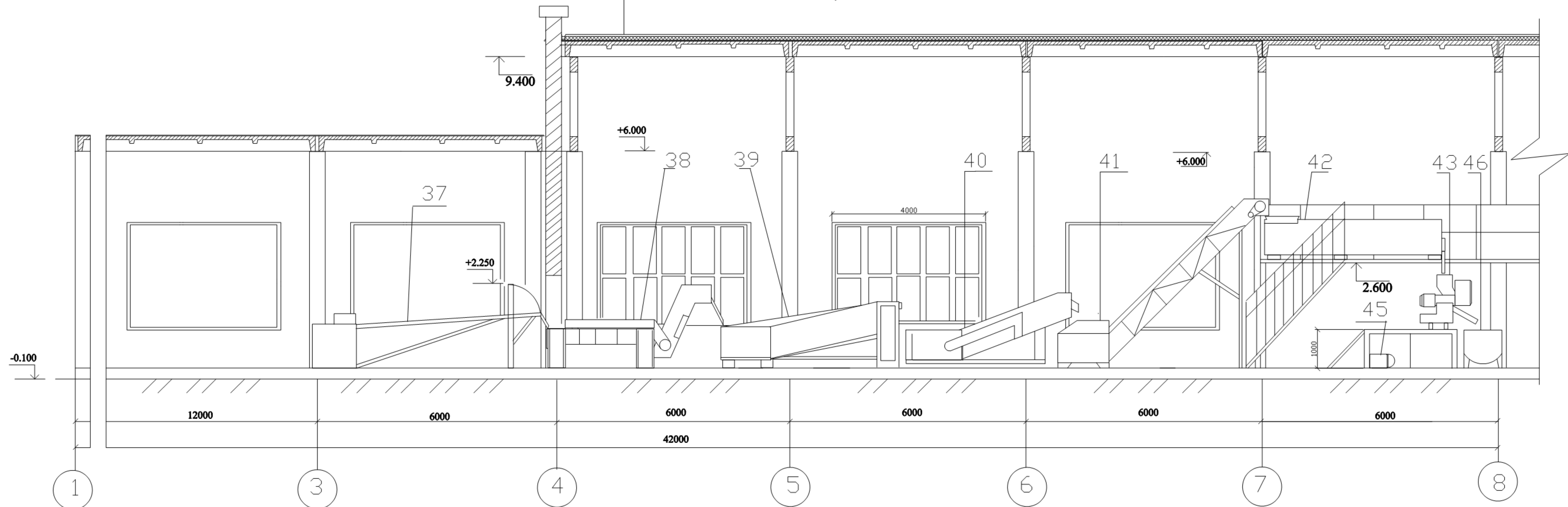
Розріз 2-2
