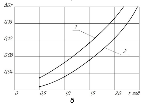
Рис. 2. Криві зносу колодки (1) і ролика (2) при звичайному (а) і вібраційному (б) деформуванні
