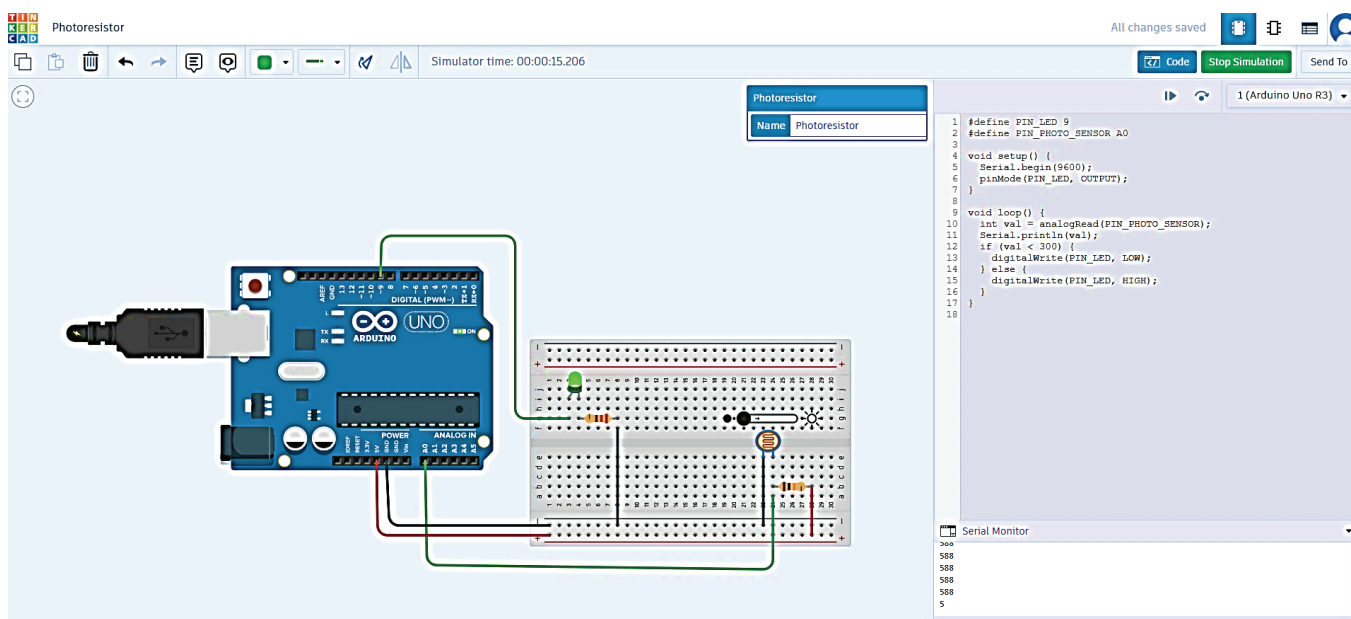
Рис. 2. Моделювання роботи датчика освітленості та програмний код у симуляторі Tinkercad
