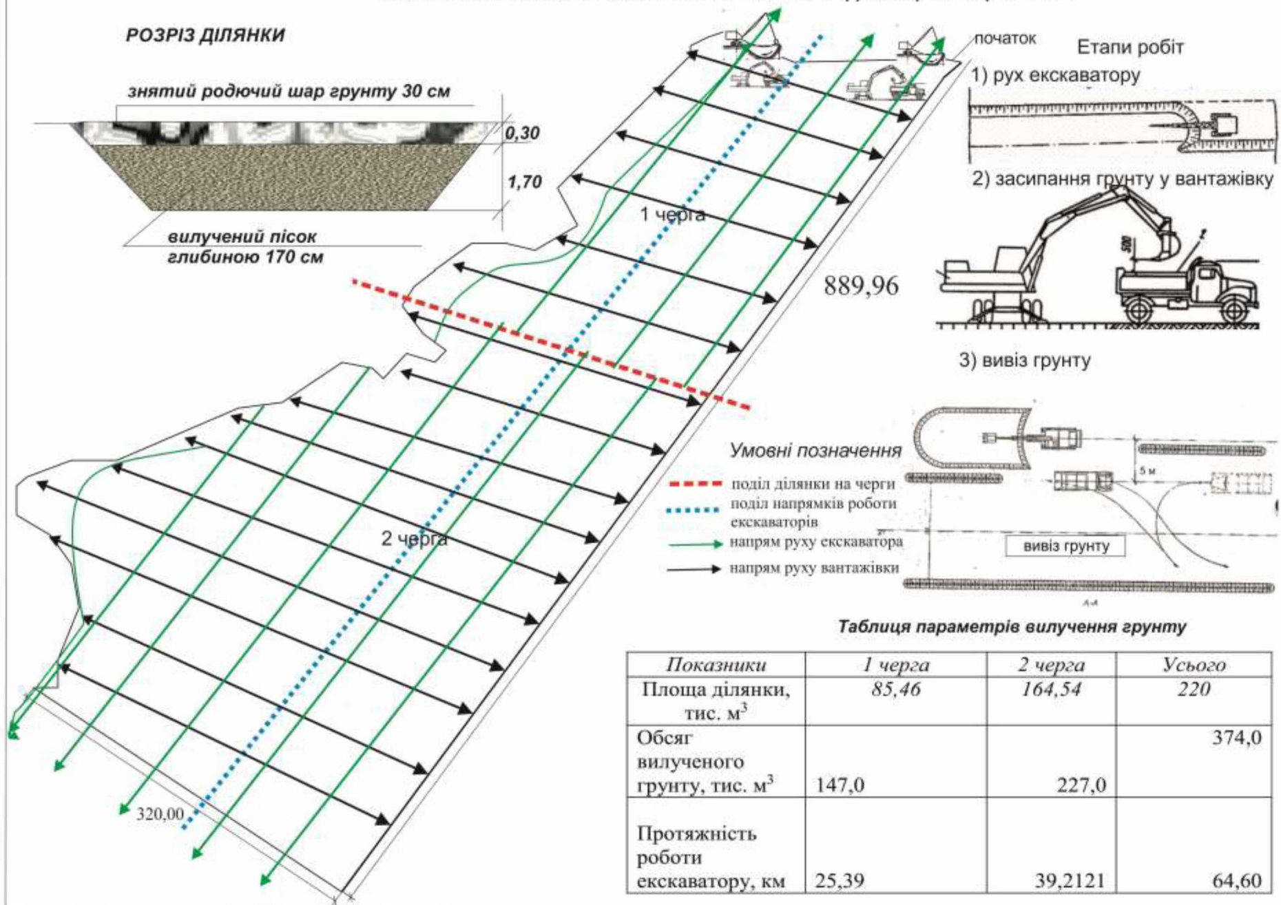
Рис.2.2 СХЕМА ВИЛУЧЕННЯ ГРУНТУ НА ГЛИБИНУ 2 м НА ДІЛЯНЦІ ПЛОЩЕЮ 22 га
