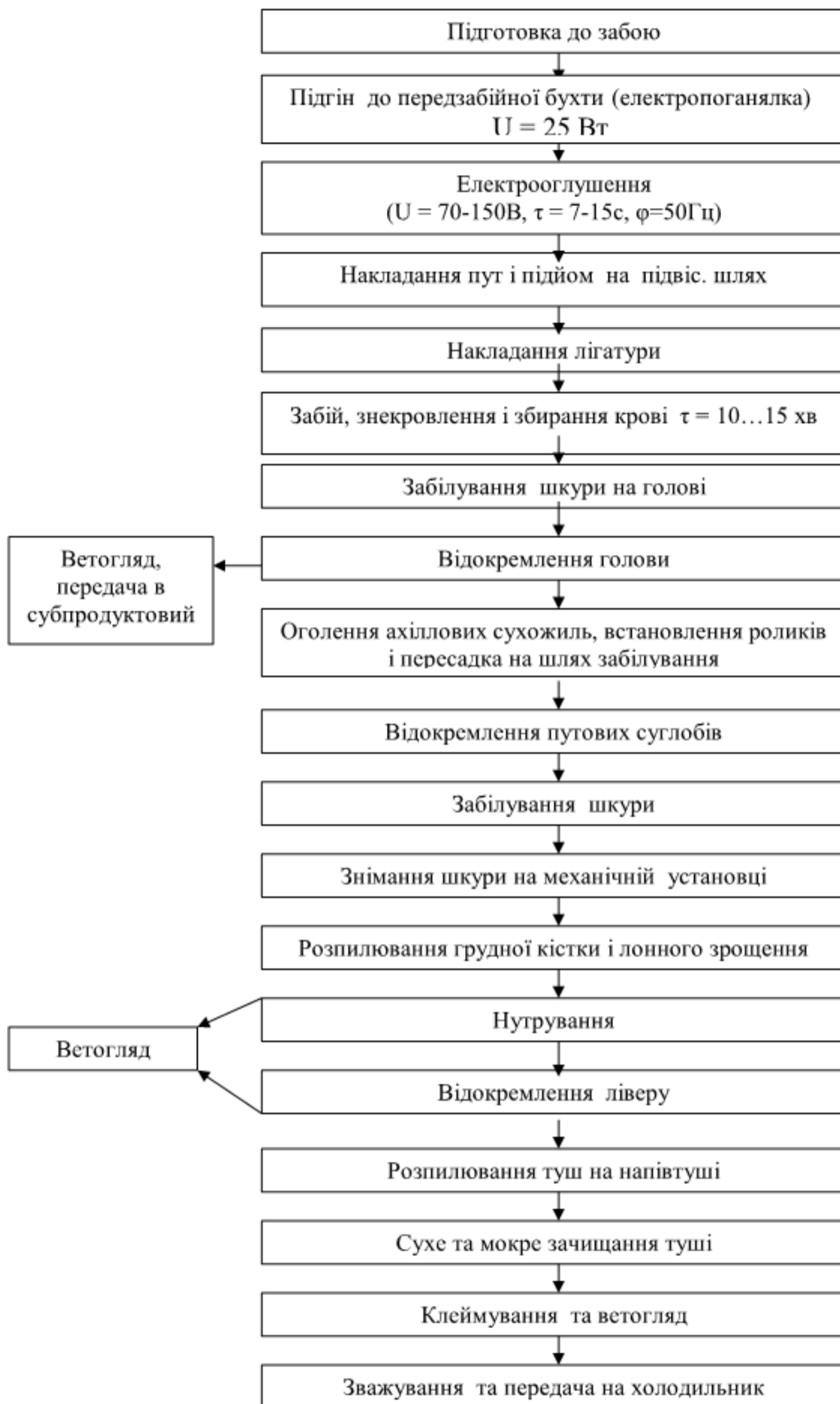
Рис. 1.1 Технологічна схема переробки врх
