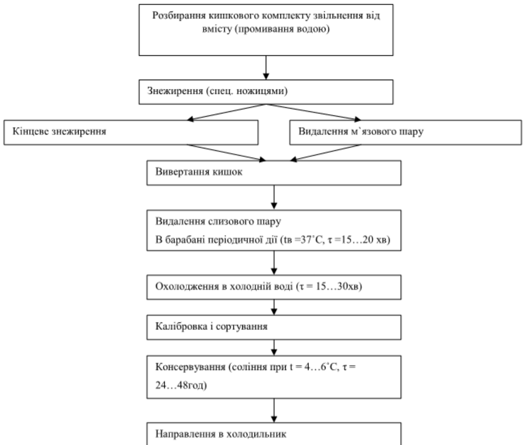
Рис. 1.6 Технологічна схема обробки кругів, синюг, прохідників ВРХ
