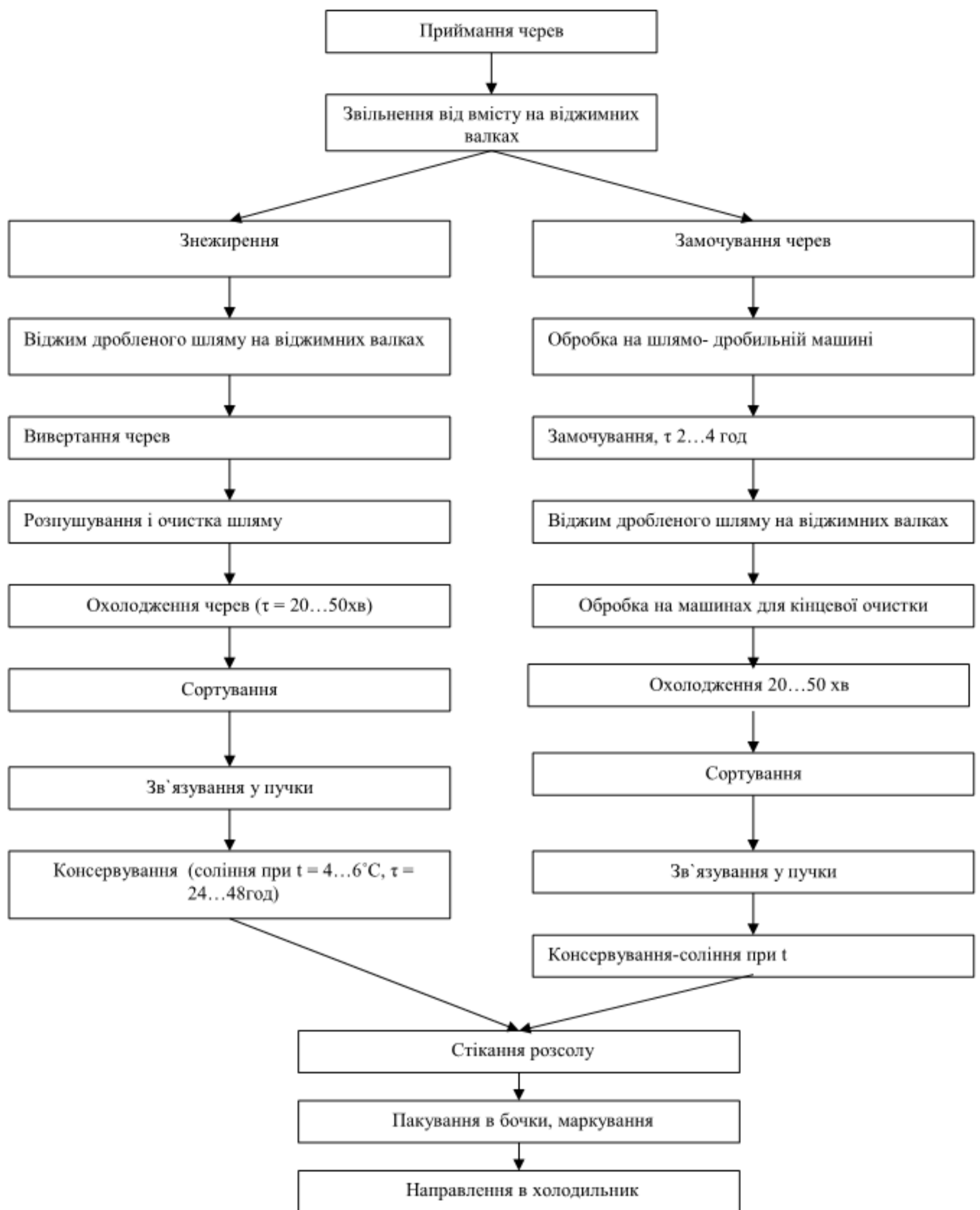
Рис. 1.5. Технологічна схема обробки кругів, свиног, прохідників ВРХ
