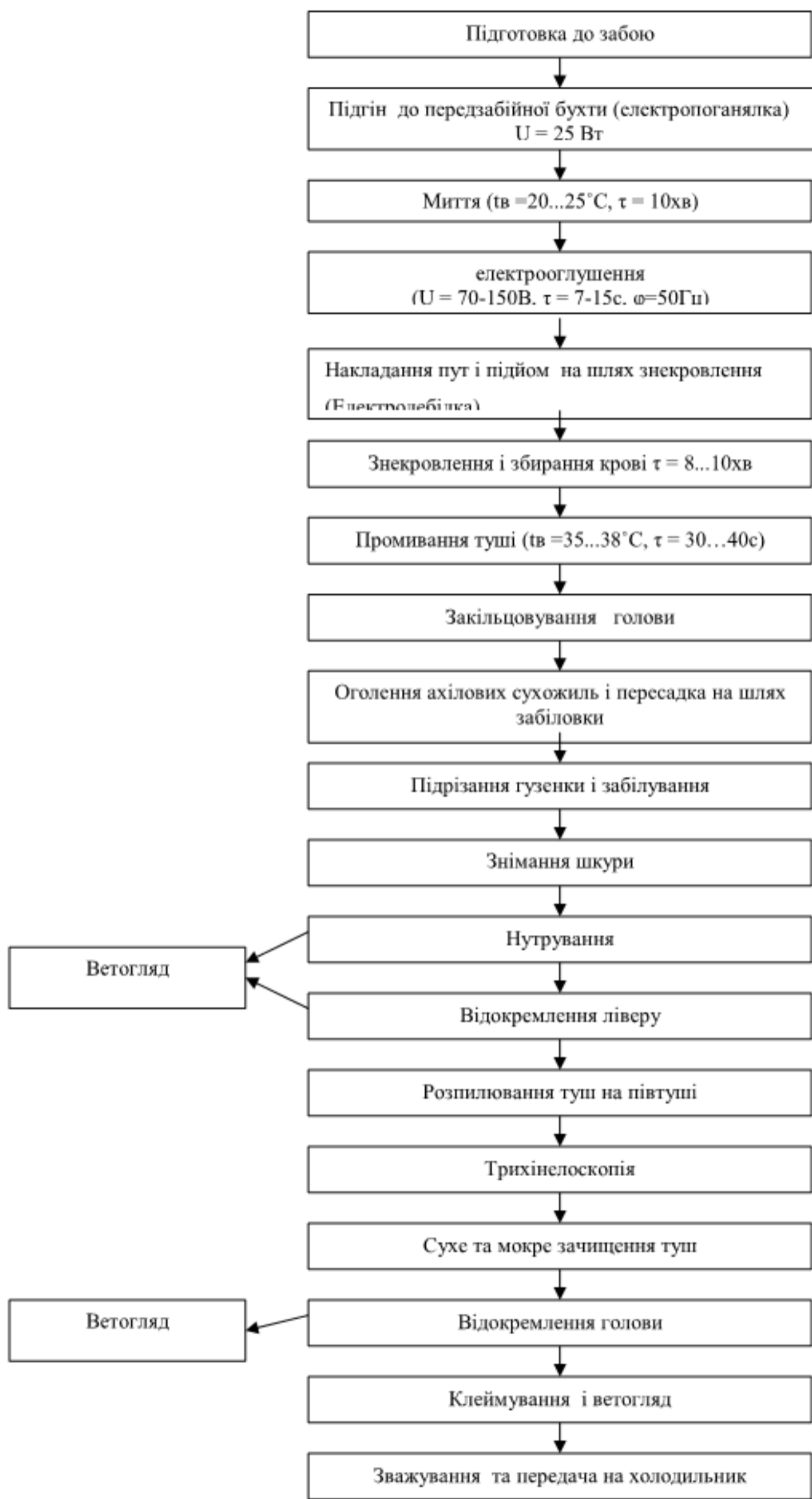
Рис. 1.2 Технологічна схема переробки свиней із зніманням шкіри
