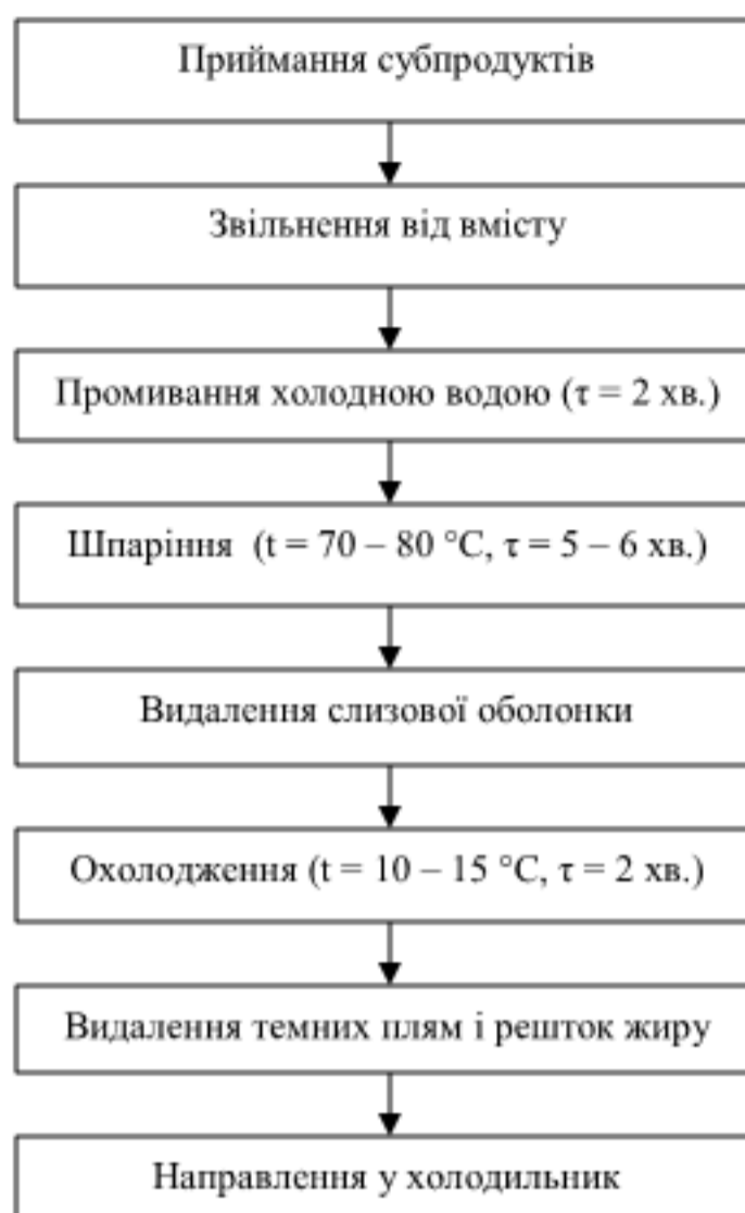
Рис. 1.7 Технологічна схема обробки слизових субпродуктів
