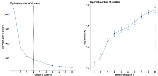
Рис. 5. Вибір оптимальної кількості кластерів методом k-means та GAP-статистикою
