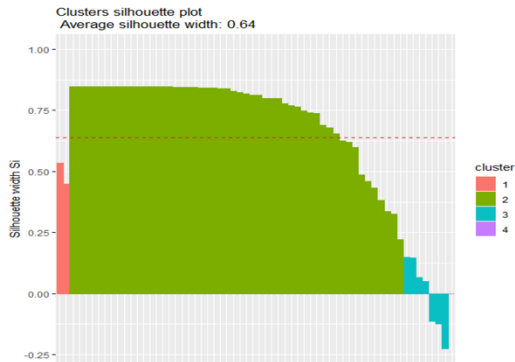
Рис. 4. Діаграма силуетів, розділених на 4 кластери
