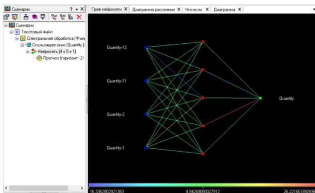
Рис. 4. Граф неймерережі
