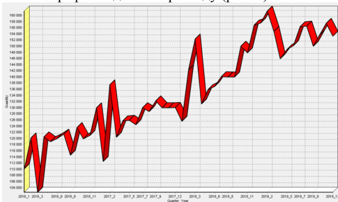
Рис. 1. Початкові дані
