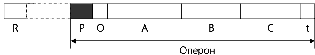
Рис. 2. Будова оперону (транскриптону) прокаріот: R – ген-регулятор; P – промотор; O – оператор; A, B, C – структурні гени; t – термінатор.
