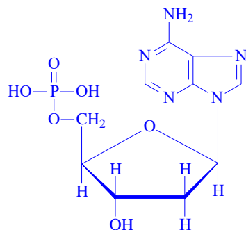
Дезоксиаденозинмонофосфорна кислота (дАМФ)
