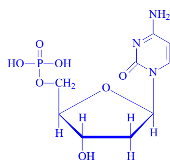
Дезоксицитидинмонофосфорна кислота (дЦМФ)
