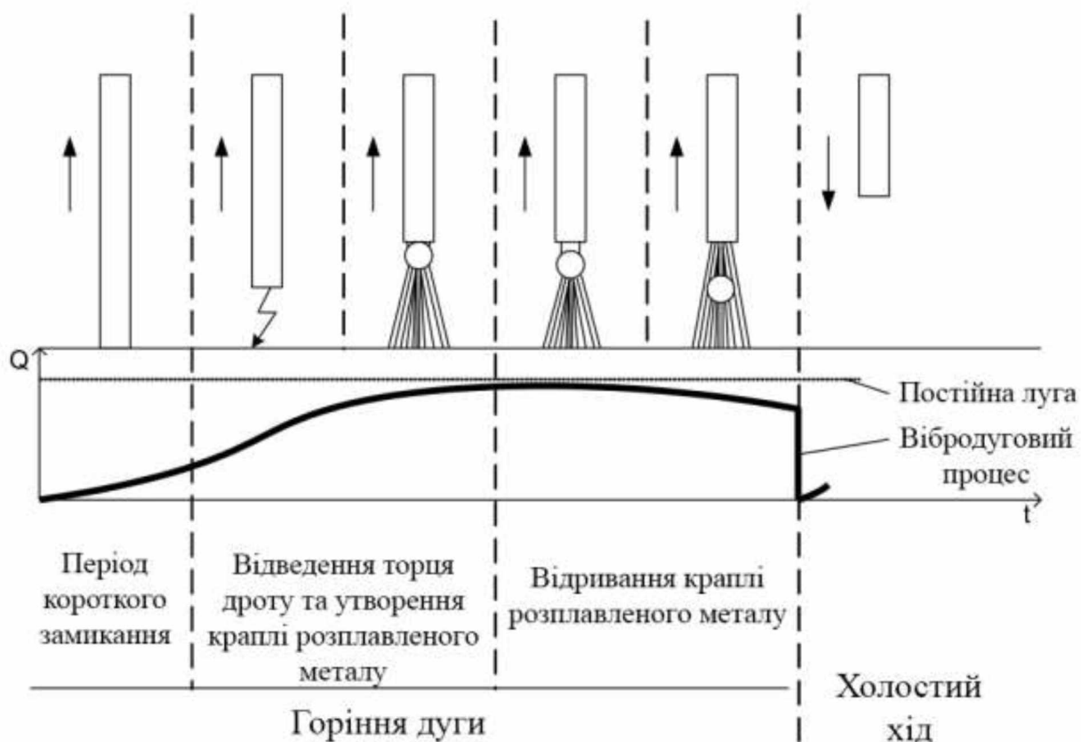
Рис. 1.6 – Схема руху дроту при вібродуговому наплавленні
