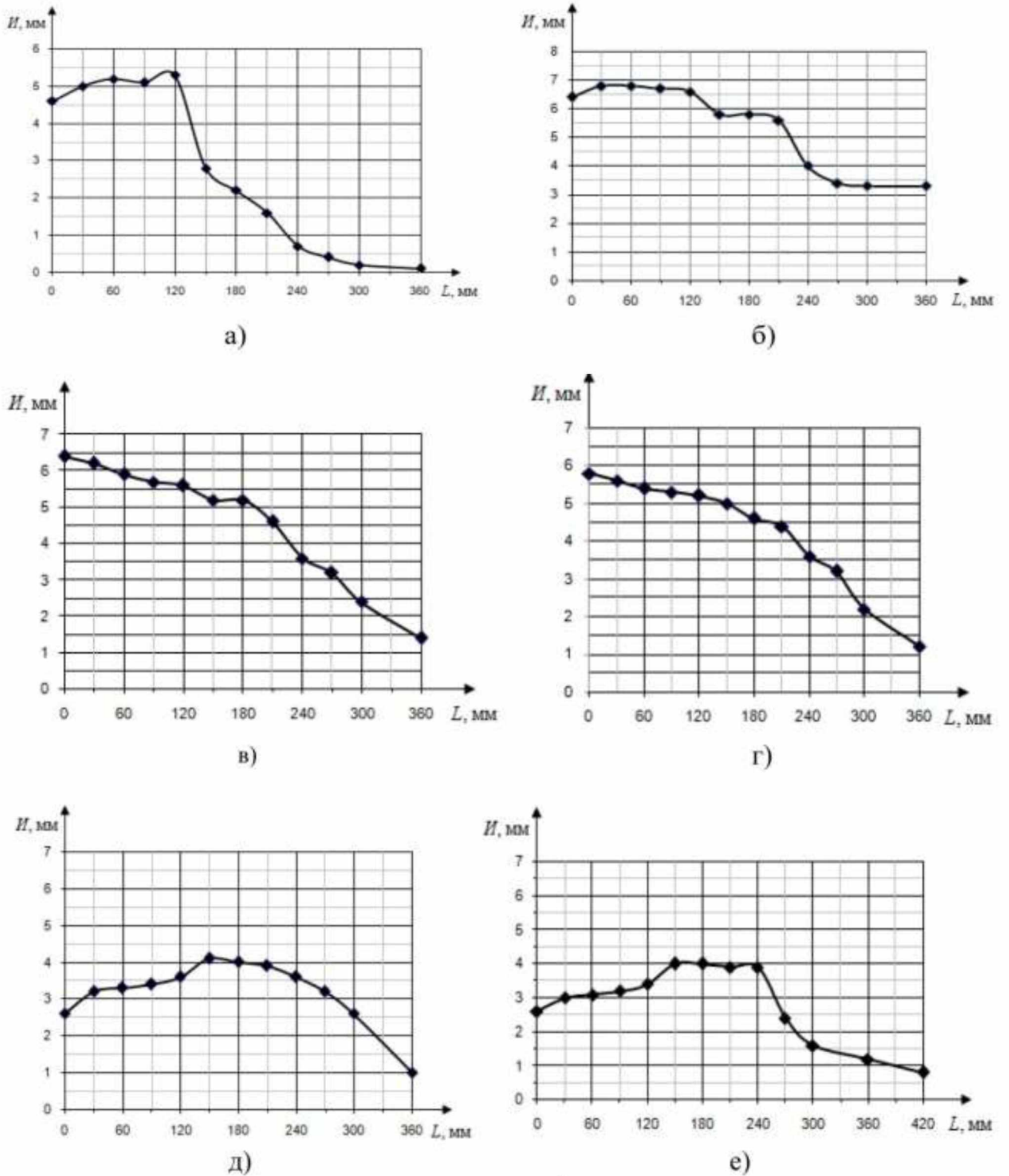
Рис. 3.10 – Характер зносу відвалів в горизонтальній площині а) – е) по лініях I–VI відповідно
