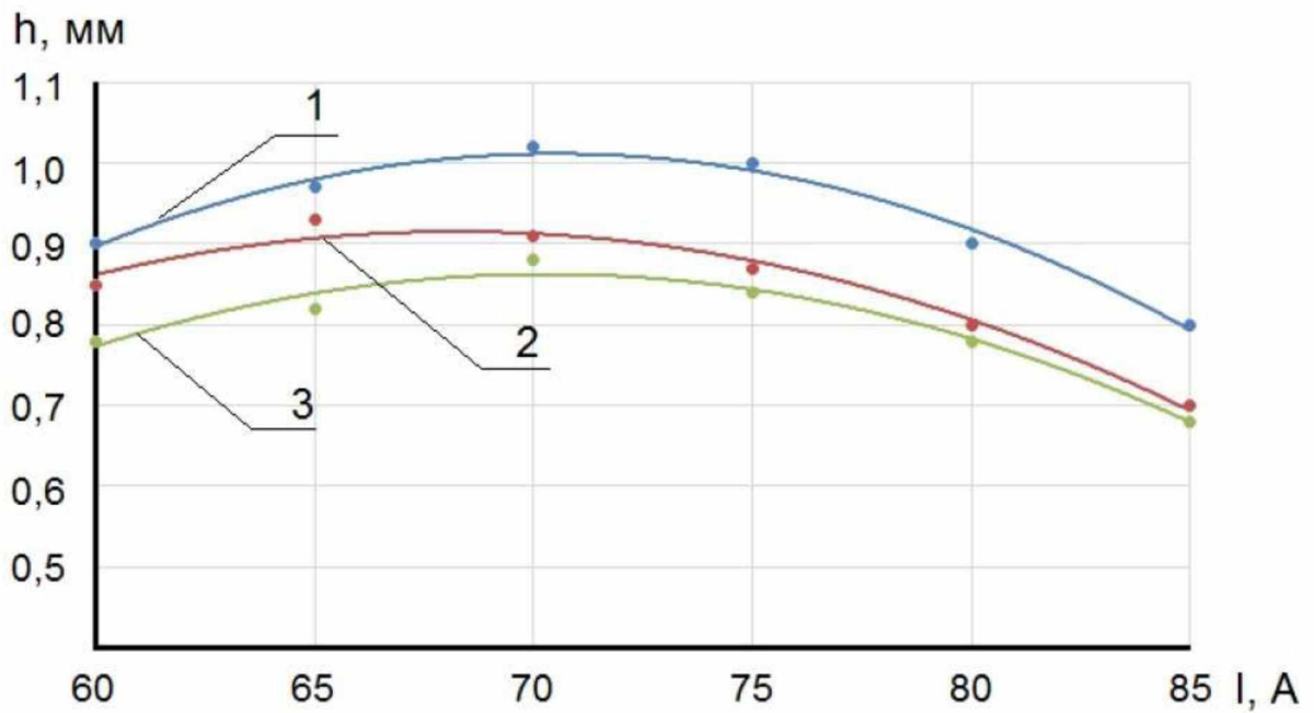
Рисунок 3.3 – Зміна товщини h металокерамічного покриття в залежності від сили струму I . Режимми КВДЗ: f = 25 Гц, A = 0,5 мм, товщина шару нанесеної пасти – 2,2 ... 2,3 мм
