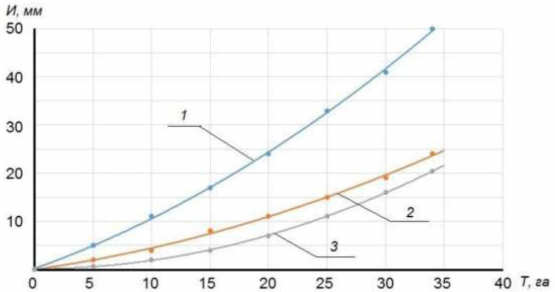
Рисунок 3.6 – Залежність зносу ( I ) носка стрічастих лап культиватора КШН-12Н від напрацювання ( T ): 1 – серійна незміцнена лапа; 2 – лапа, зміцнена КВДЗ з лицьового боку; 3 – лапа, зміцнена КВДЗ з тильного боку
