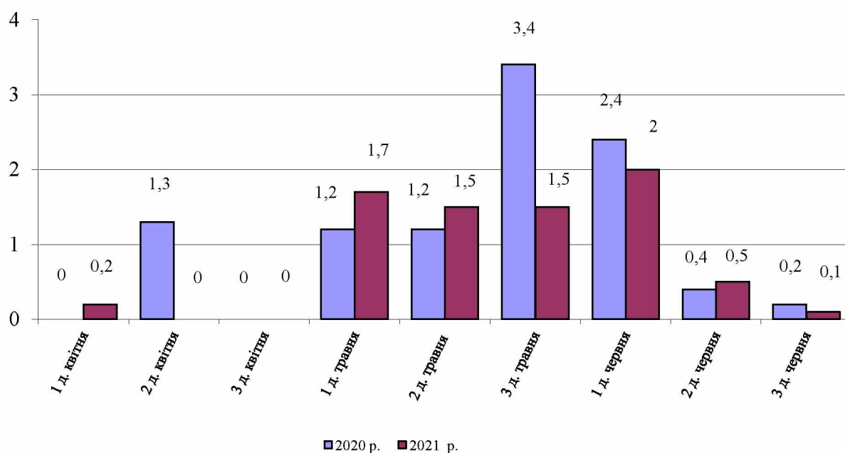
Рис. 3.3. Гідротермічний коефіцієнт під час досліджень
