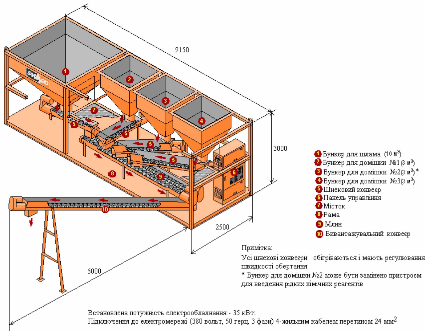
Рисунок 3.3 - Блок нейтралізації шламу фірми "Swaco"
