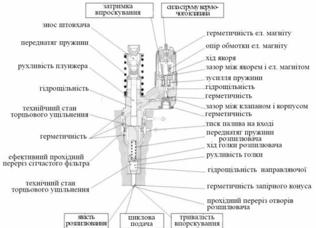
Рисунок 3.1 – Найбільш значущі структурні і діагностичні (в рамці) параметри насос-форсунки 0414701019 фірми Bosch
