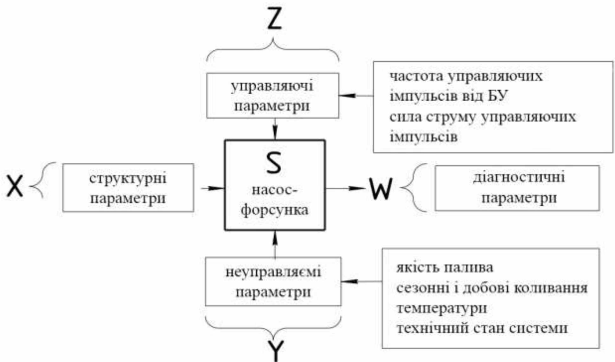
Рисунок 3.2 – Інформаційна модель функціонування насос-форсунки
