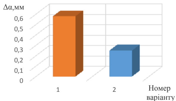
Рис. 4 – Діаграма зміни товщини \Delta a леза дисків Ø350 мм при стендових випробуваннях: 1 – нові диски зі сталі 65Г; 2 – відновлені приварюванням сегментів зі сталі 45 з наплавленням сормайтотом і вібраційним зміцненням
