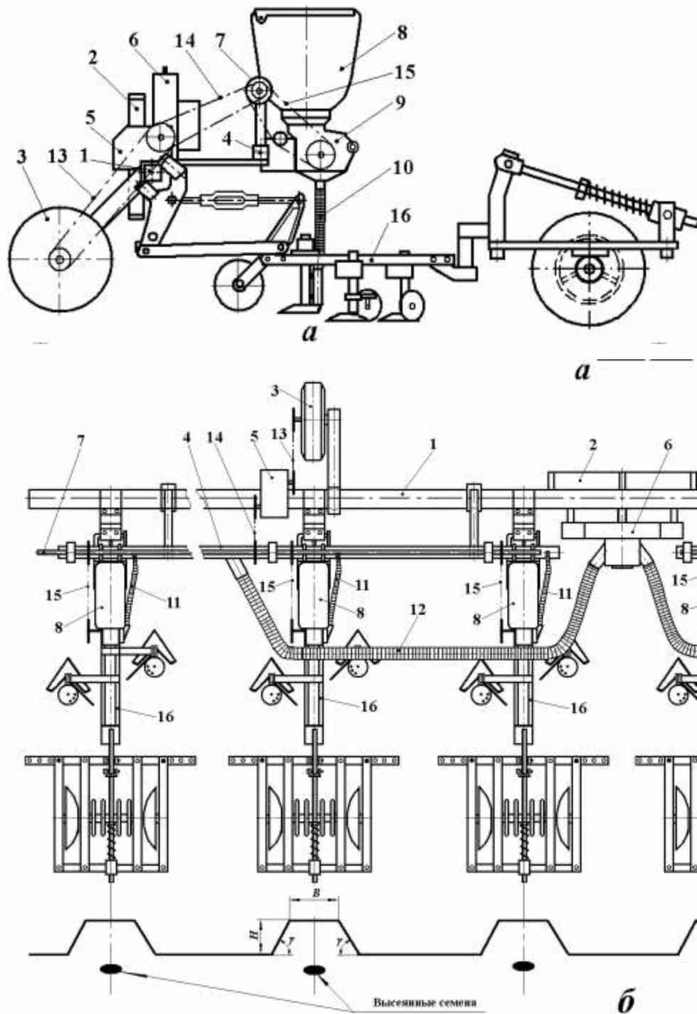
Рисунок 2.1 – Гребенева сівалка: а - вид збоку; б - вид зверху
