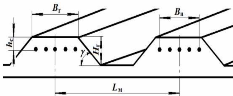
Рисунок 1.2 – Розташування насіння, висіяного смугами в гребені ґрунту: B_n – ширина смуги посіву
