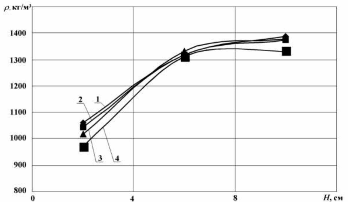
Рисунок 3.7 – Залежності щільності ґрунту по висоті гребеня від зусилля пружини котка-гребенеутворювача при \alpha_{сд} = 20^\circ , V_C = 1,6 м/с
