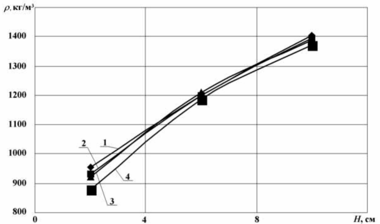
Рисунок 3.6 – Залежність щільності ґрунту по висоті гребеня від зусилля пружини котка-гребенеутворювача при \alpha_{сд} = 10^\circ , V_C = 1,6 м/с
