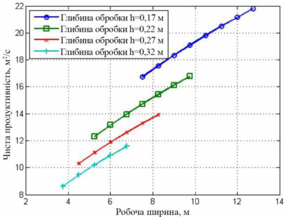
Рисунок 3.3 – Залежність продуктивності від ширини захвату при різній глибині обробки
