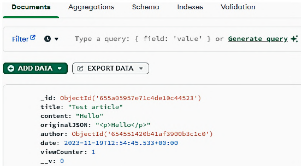
Рисунок 3.10 – Приклад документу MongoDB
