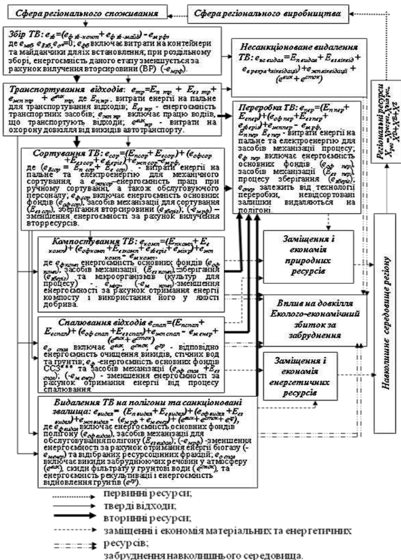
Рис.1 – Балансова схема життєвого циклу твердих відходів регіону
