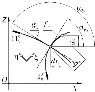
Рис. 3. Сліди координатних поверхонь системи НΞУ на площині XOZ
