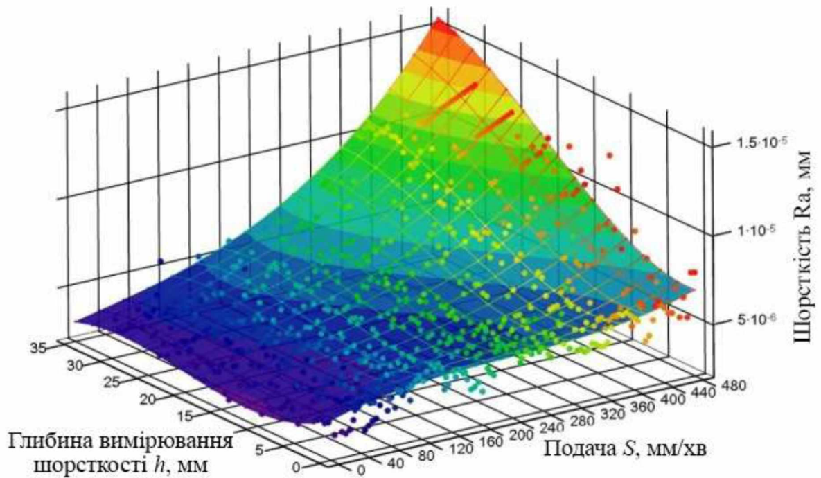
Рисунок 3.7 – Двухфакторная модель формування шорсткості поверхні різу при вимірюванні шорсткості вздовж розтину різу
