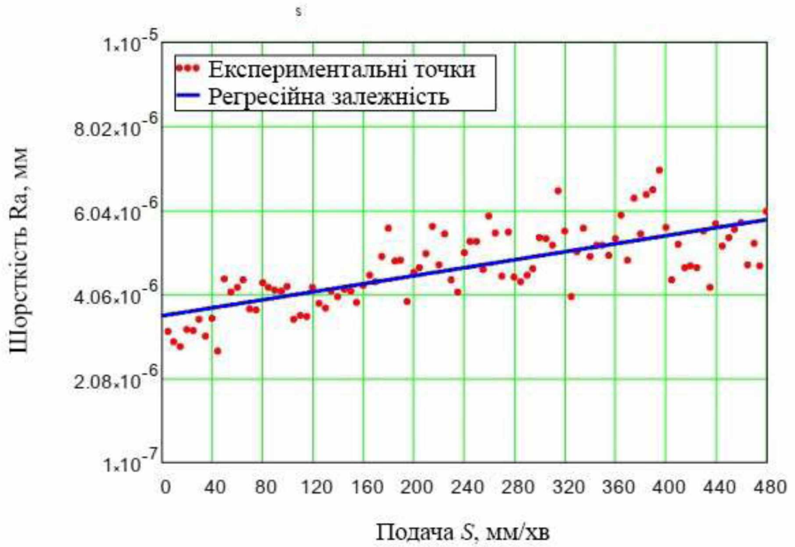
Рисунок 3.6 – Формування шорсткості поверхні різу при вимірюванні поперек перетину різу
