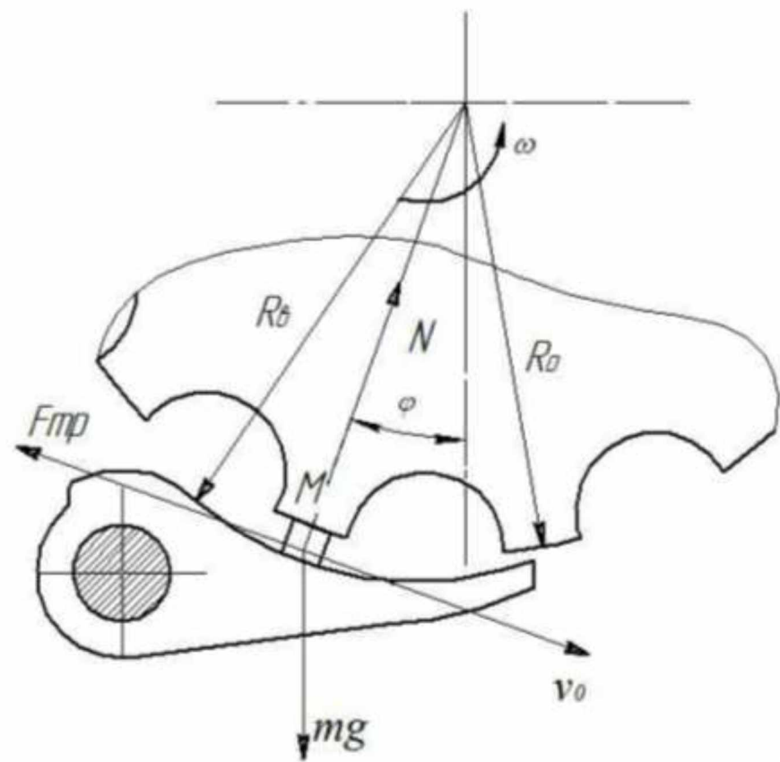
Рисунок 3.4 – Схема для визначення початкової швидкості насіння на клапані
