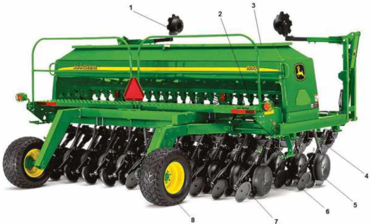
Рисунок 1.6 – Сівалка John Deer 1590: 1 - маркер; 2 - висіваючий апарат; 3 - бункер; 4 підвіска; 5 - копіювальне колесо; 6 - зароблююче колесо; 7 - колесо для накочування; 8 – привідне колесо
