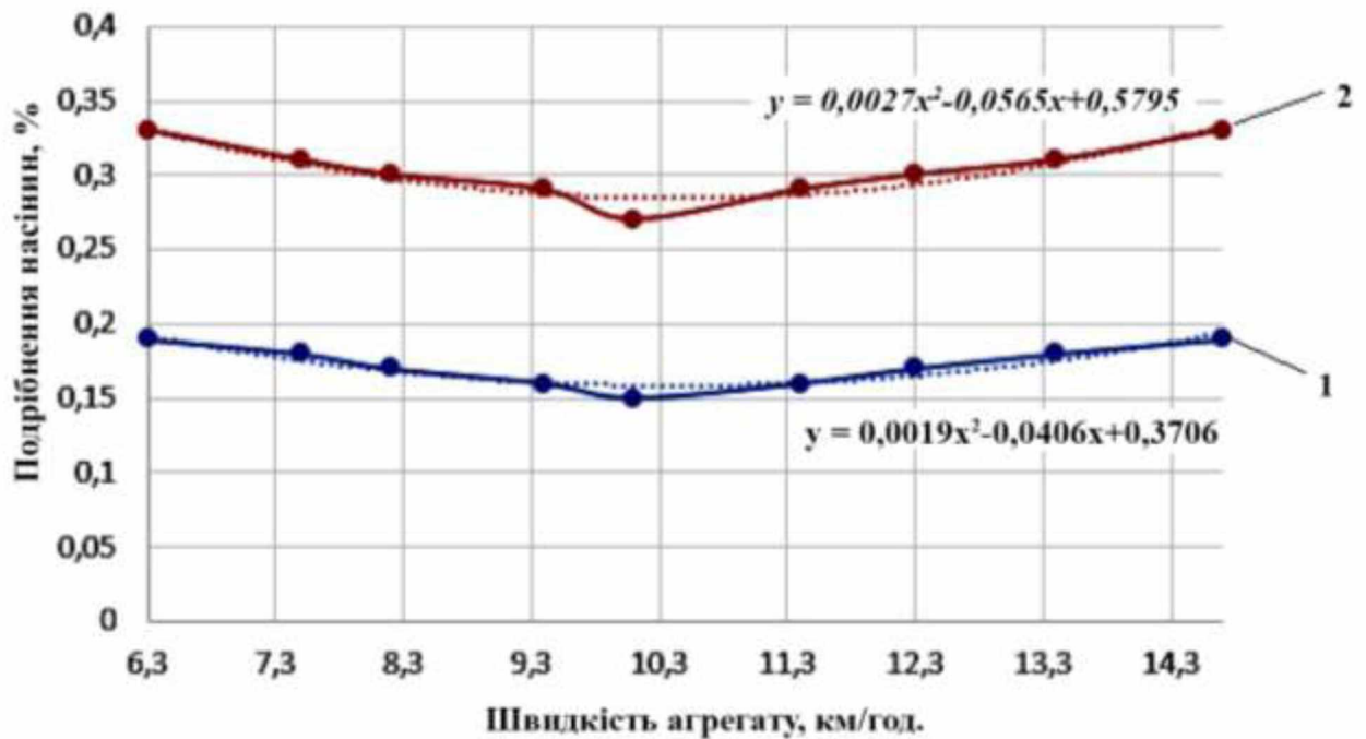
Рисунок 3.9 – Графіки залежності дроблення насіння зернових культур від швидкості агрегату; 1 - експериментальна сівалка, 2 - серійна сівалка
