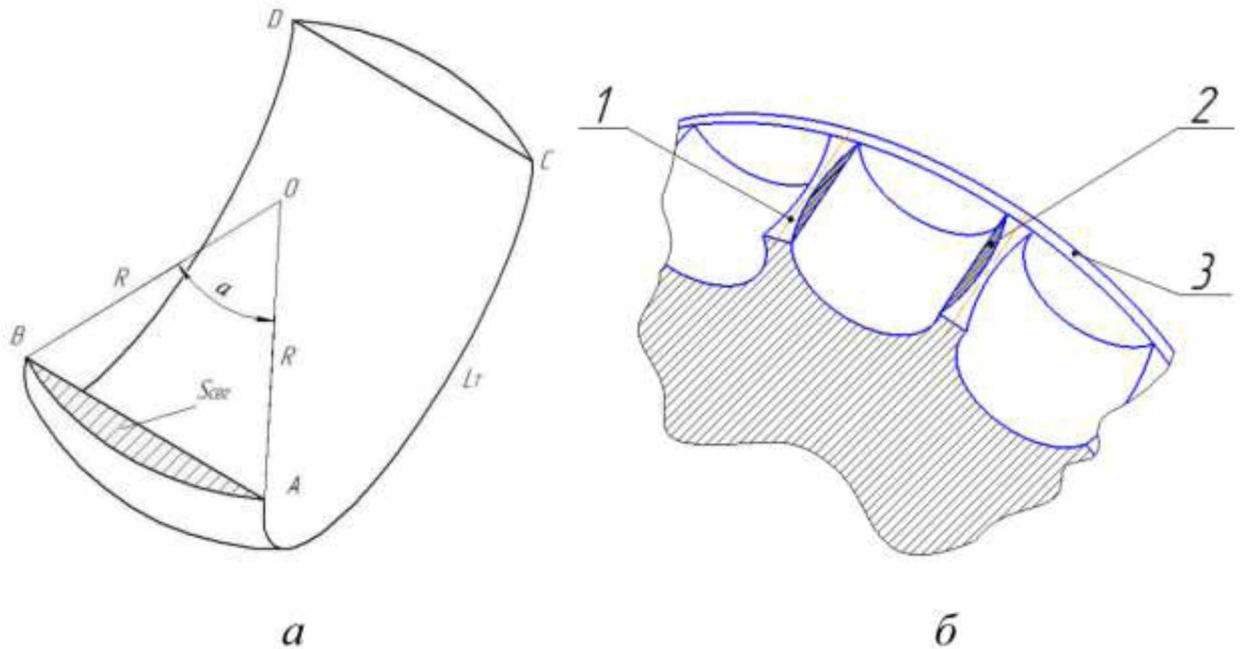
Рисунок 3.2 – Схема секції чотирьохсекційної котушки, жолобки якої виконані у формі частини тора:
