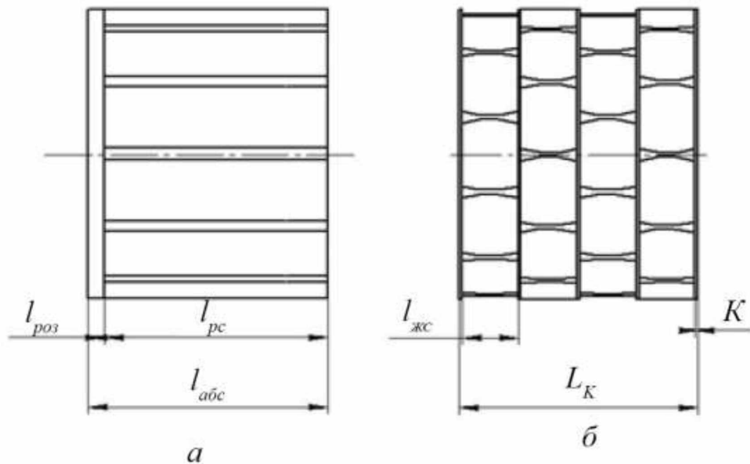
Рисунок 3.3 – Схема котушок для визначення довжини одного жолобка чотирьохсекційної котушки: а) стандартна котушка; б) чотирьохсекційна котушка, жолобки якої виконані у формі частини поверхні обертання тора
