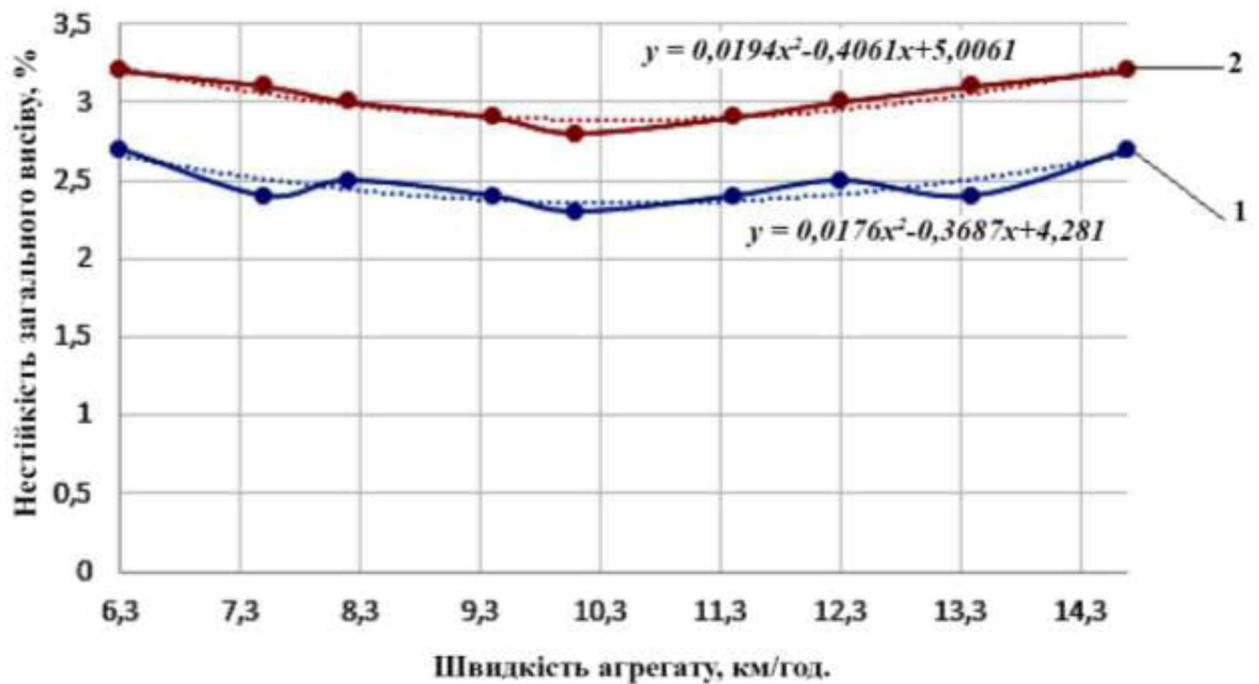
Рисунок 3.8 – Графіки залежності нестійкості загальної норми висіву від швидкості агрегату; 1 – експериментальна сівалка, 2 - серійна сівалка
