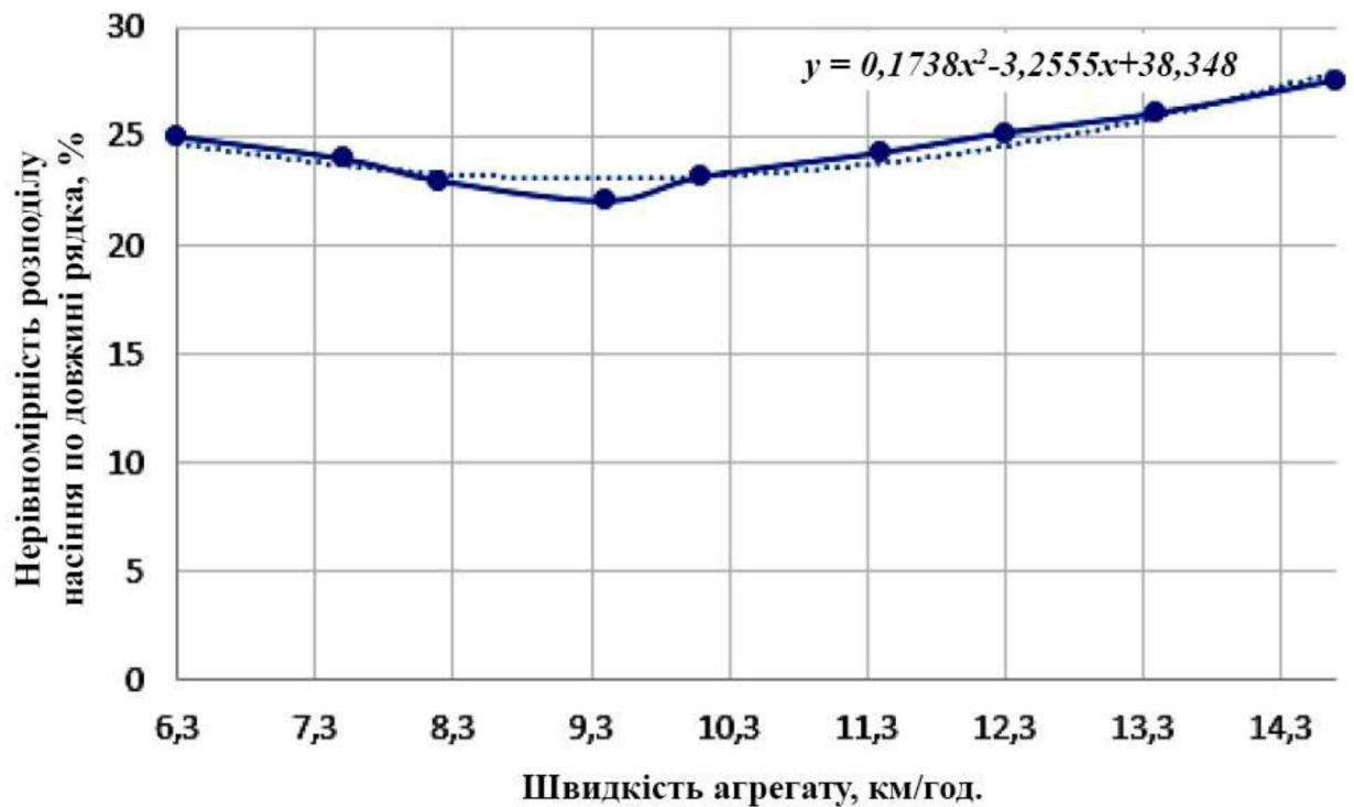
Рисунок 3.7 – Графіки залежності нерівномірності розподілу насіння ( v ) зернових культур по довжині рядка від швидкості руху агрегату ( u )
