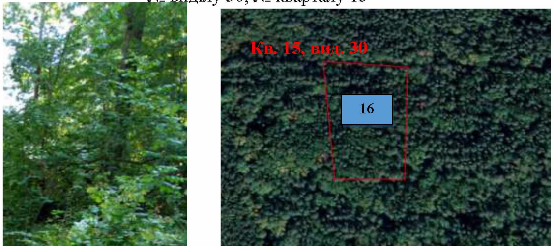
Рис. 43 - Схема розташування місця дослідження ґрунтового розрізу у Варвинському лісництві (розріз 16)
