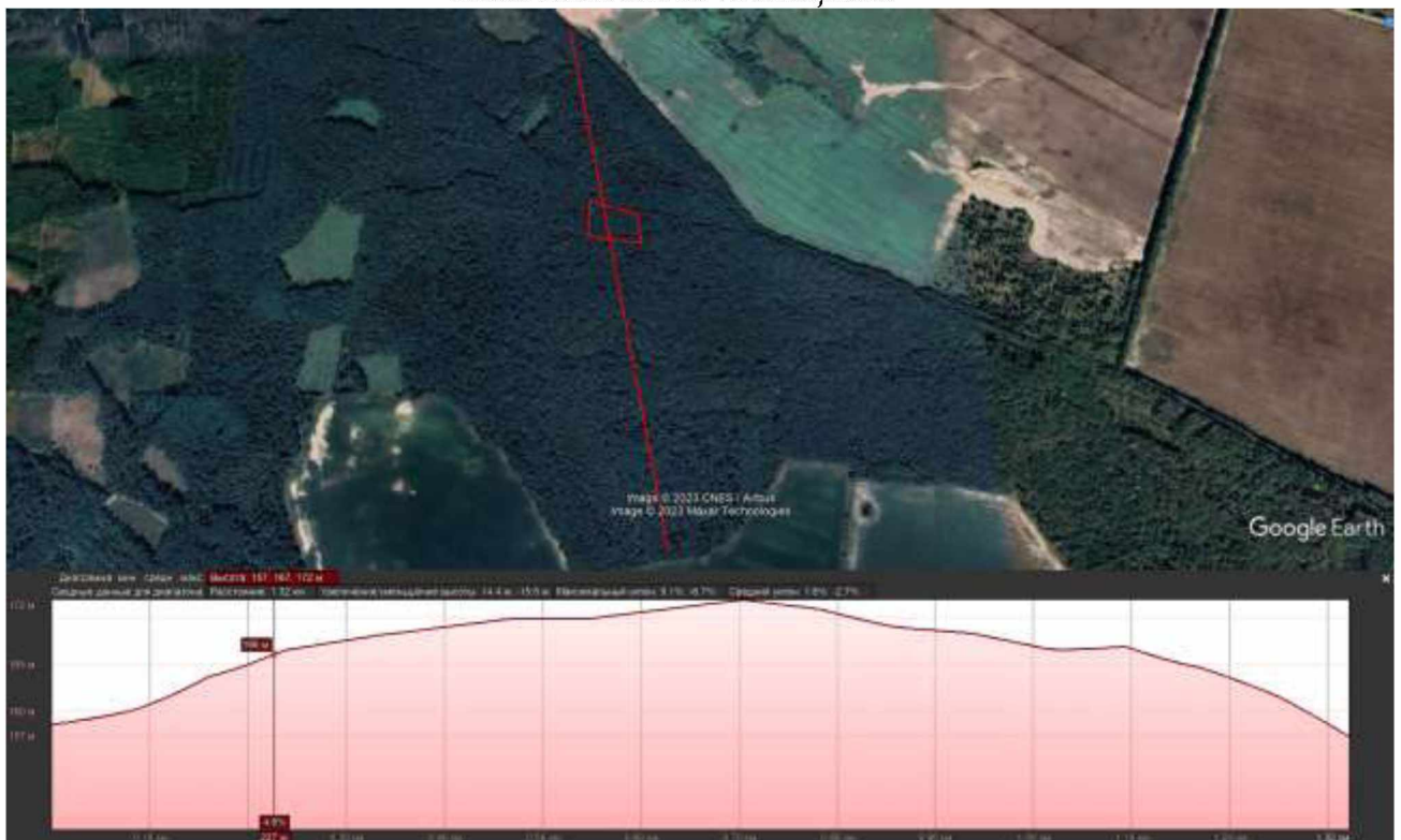
Рис. 23 - Продольний профіль місцевості в районі розташування Жадьківського лісництва
