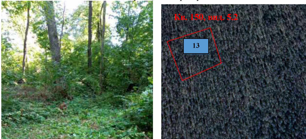
Рис. 40 - Схема розташування місця дослідження ґрунтового розрізу у Прилуцькому лісництві (розріз 13)
