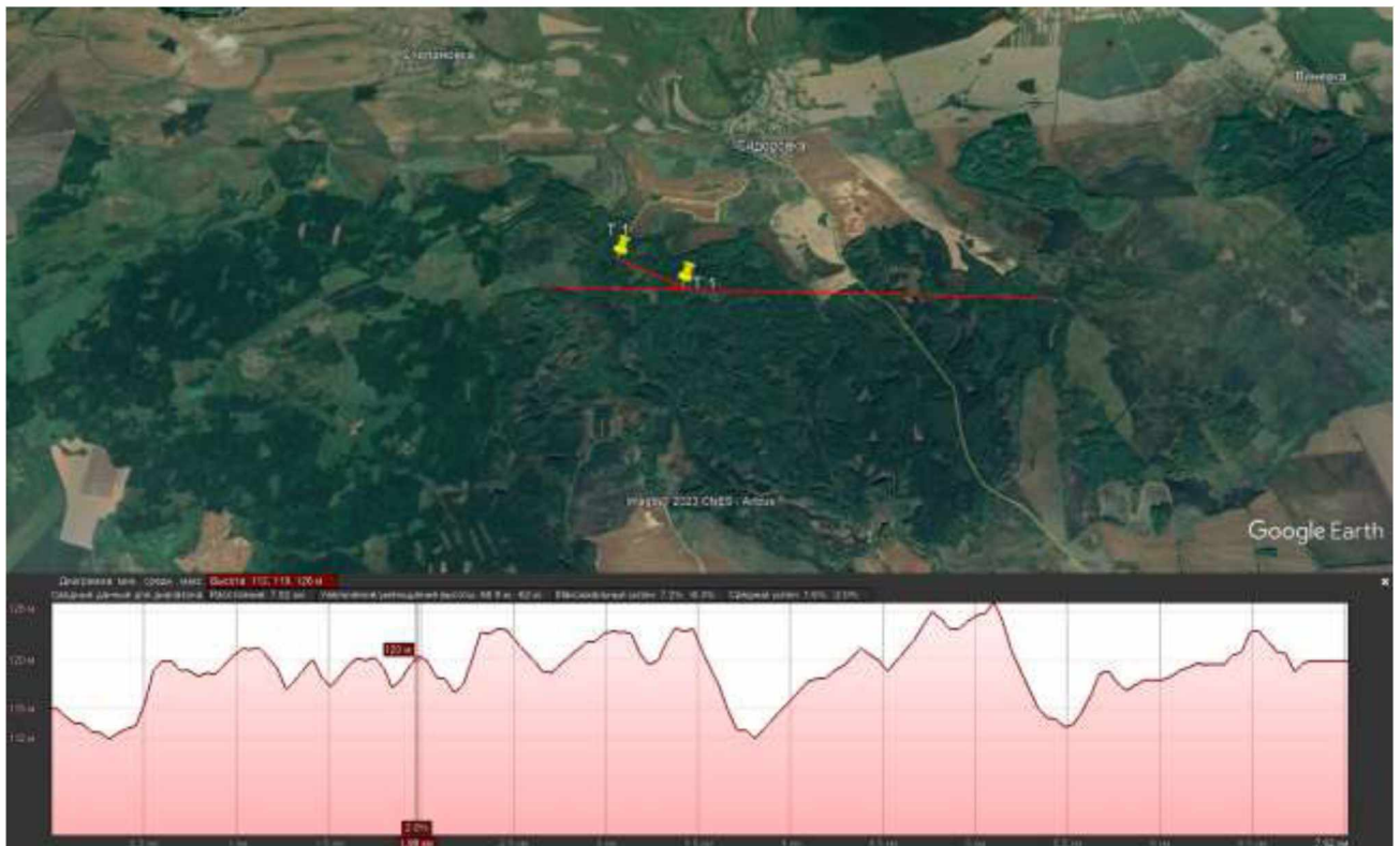
Рис. 2 - Поперечний профіль місцевості в районі розташування Берестовського лісництва
