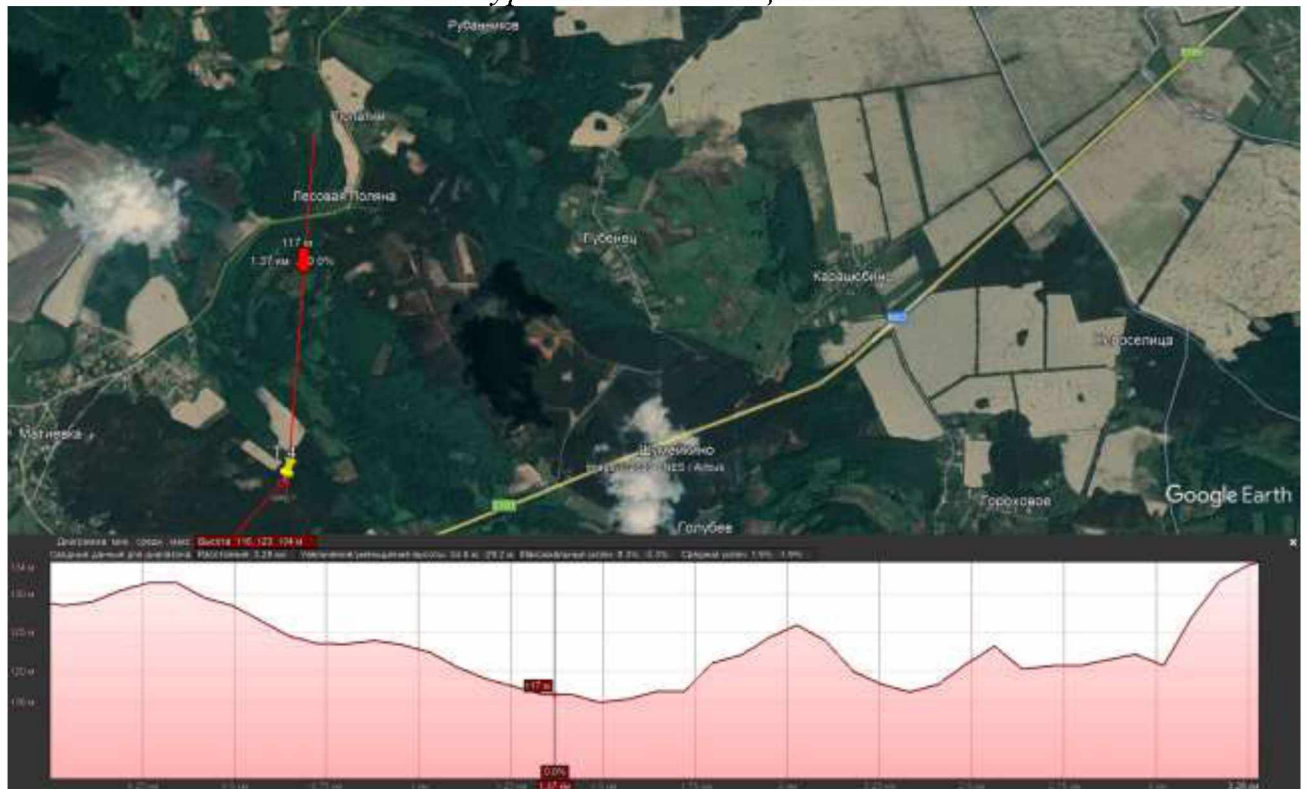
Рис. 7 - Продольний профіль місцевості в районі розташування Батуринського лісництва
