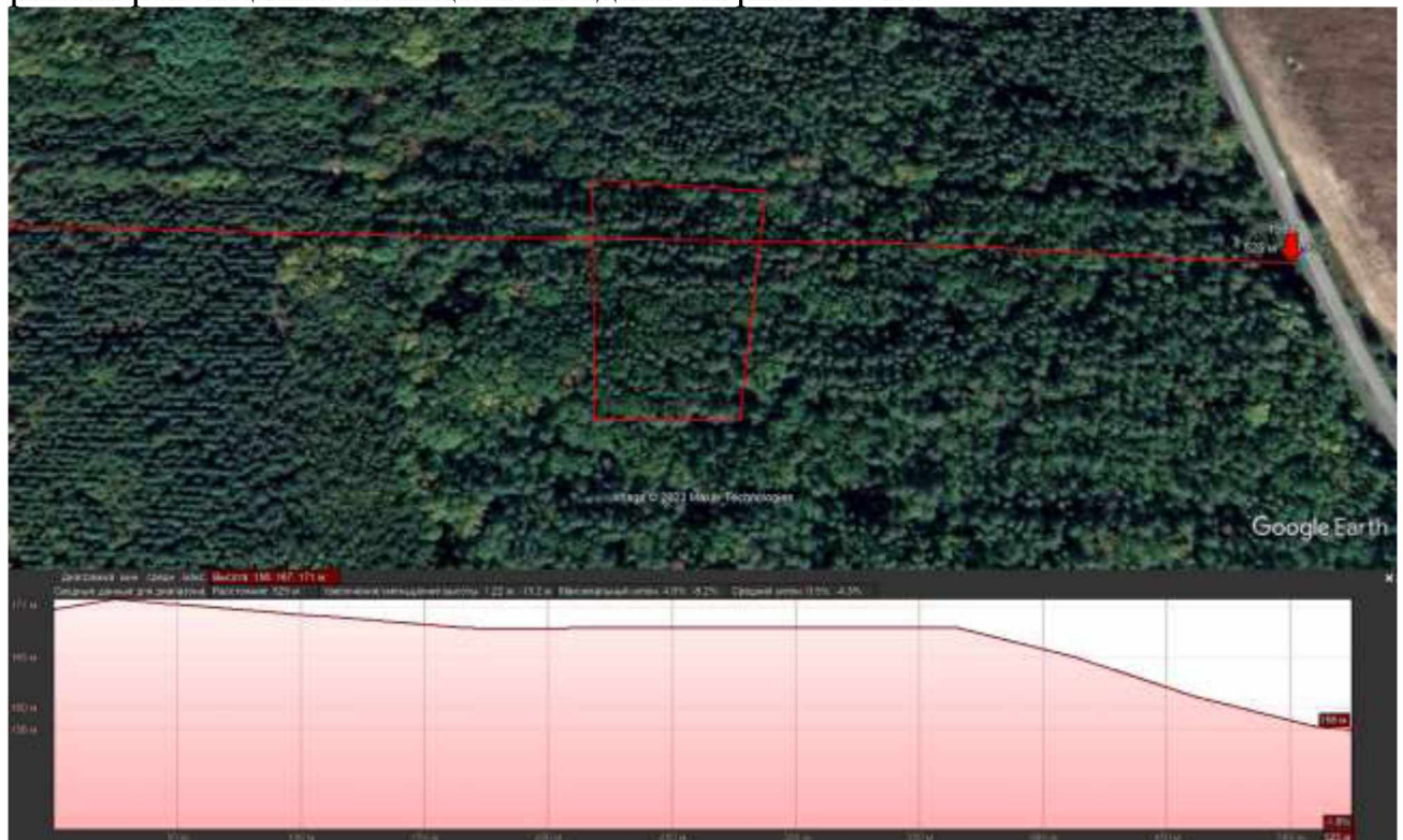
Рис. 24- Поперечний профіль місцевості в районі розташування Кам'янського лісництва
