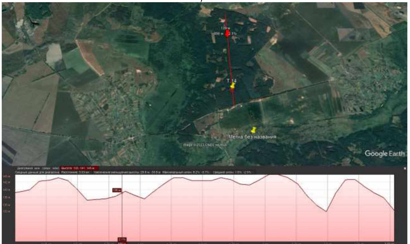
Рис. 18 - Поперечний профіль місцевості в районі розташування Ічнянського лісництва
