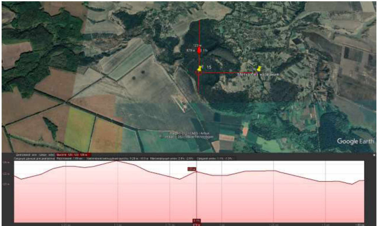
Рис. 21 - Продольний профіль місцевості в районі розташування Прилуцького лісництва
