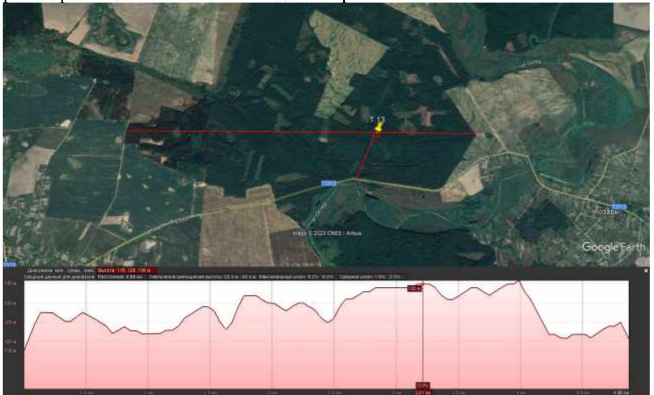
Рис. 14 - Поперечний профіль місцевості в районі розташування Іржавського лісництва
