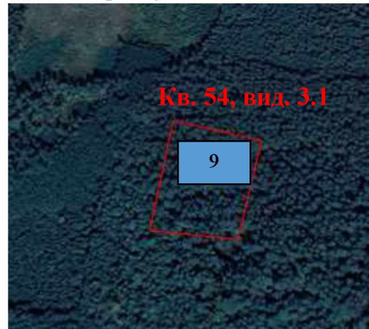
Рис. 36 - Схема розташування місця дослідження ґрунтового розрізу у Іржавському лісництві (розріз 9)
