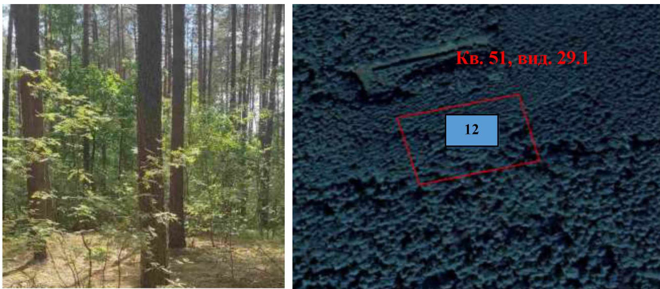
Рис. 39 - Схема розташування місця дослідження ґрунтового розрізу у Ічнянському лісництві (розріз 12)
