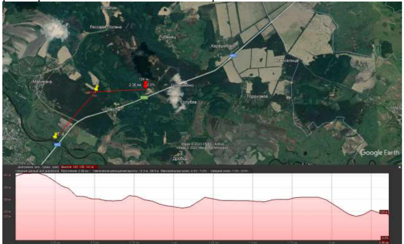
Рис. 6 - Поперечний профіль місцевості в районі розташування Батуринського лісництва
