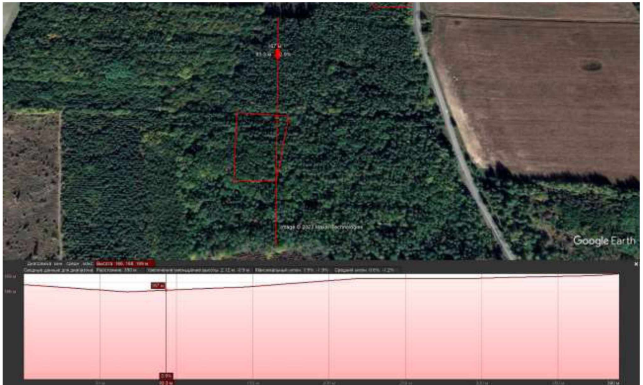
Рис. 25 - Продольний профіль місцевості в районі розташування Кам'янського лісництва
