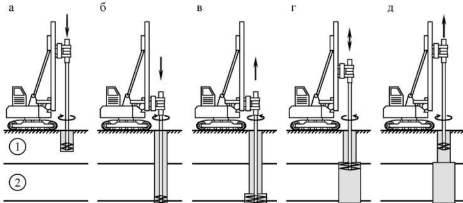
Рис. 2. Технологія влаштування розширеного ґрунтоцементного елементу у слабких ґрунтах: а-б) занурення бурозмішувача в ґрунтову основу зі складеними ножами; в) розкладання ножів шляхом зворотного обертання штанги; г) влаштування розширеного ґрунтоцементного елементу у слабкому шарі; д) складання ножа та підйом штанги; 1 – несучий шар ґрунту; 2 – слабкий шар ґрунту
