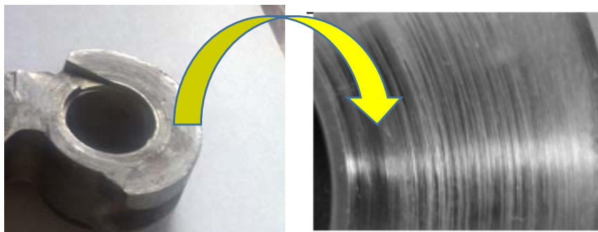
Рисунок 1 – Зовнішній вигляд втулок із гідроабразивним спрацюванням торців
