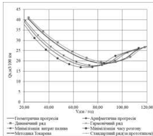
Рисунок 2 – Паливно-економічна характеристика автомобіля
