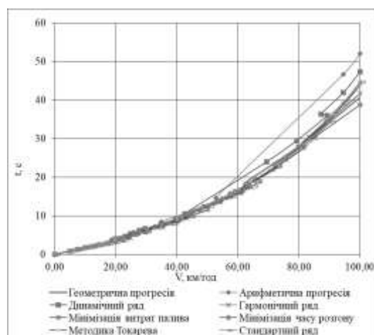
Рисунок 4 – Залежність часу розганяння від швидкості автомобіля
