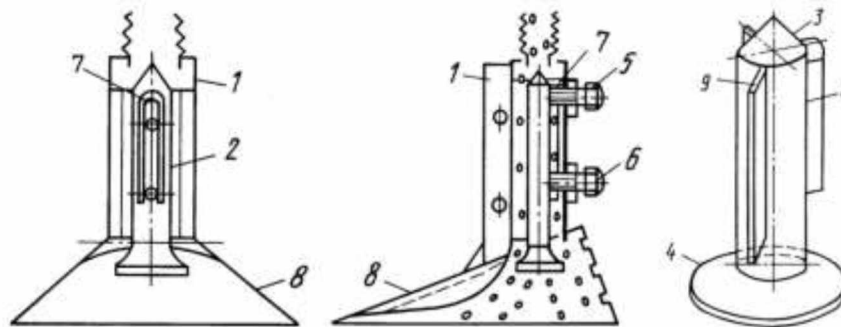
Рисунок 1.4 – Леміш для розкидного посіву: 1 - стійка-насіннєпровід; 2 - шток; 3 - конусна частина штока з прямолінійною твірною; 4 - криволінійна твірна штока; 5,6 - регулювальні болти; 7 - відбивач; 8 - стрілчаста лапа; 9 - розсікачі насіння
