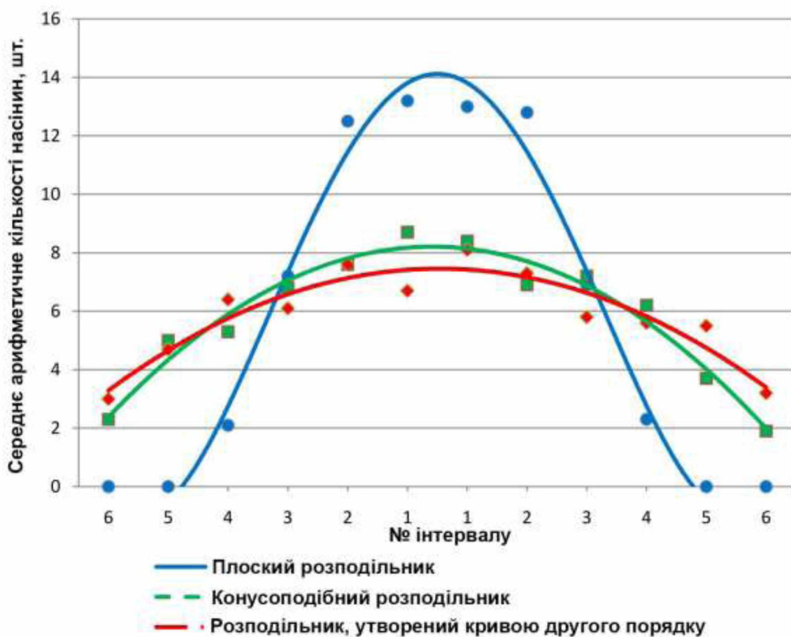
Рисунок 3.7 – Діаграма рівномірності розподілу насіння по ширині засівальної смуги в залежності від форми поверхні розподільника
