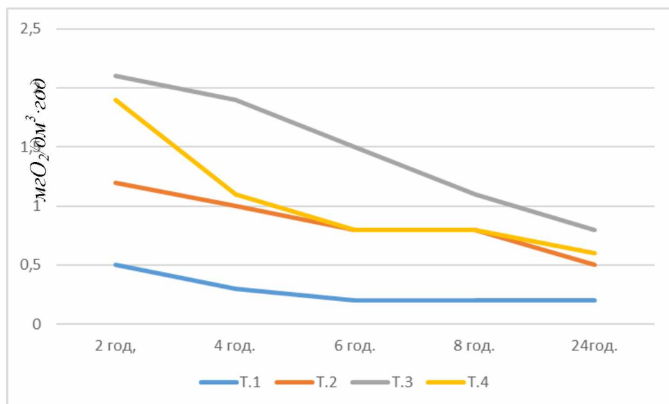
Рис. 4.2. Динаміка валової первинної продукції ( P_v ) р. Ворскла у межах м. Полтава
