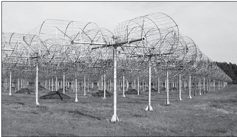
Антенна решітка радіотелескопу УРАН-2 (с. Василівка Полтавського району)
