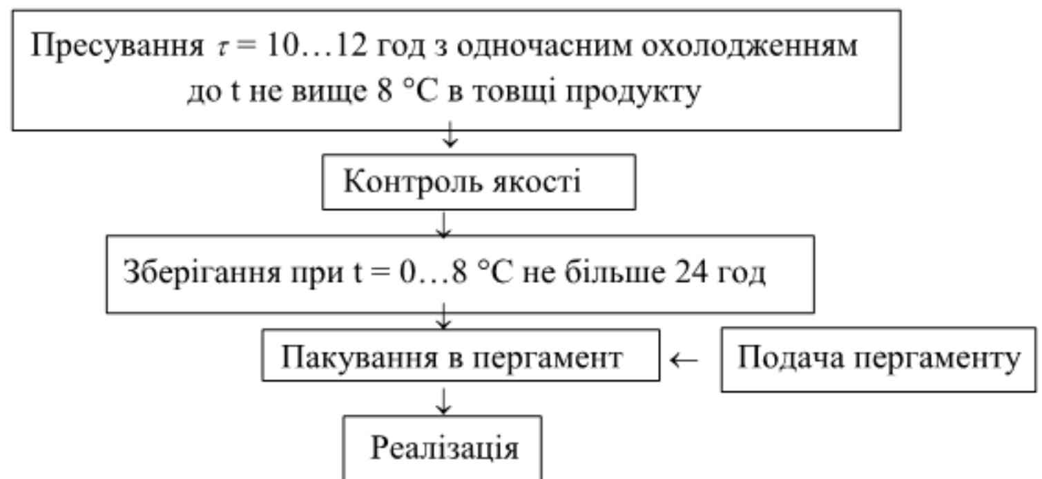
Рисунок А.3 - Технологічна схема виробництва копчено-вареного балику в оболонці
