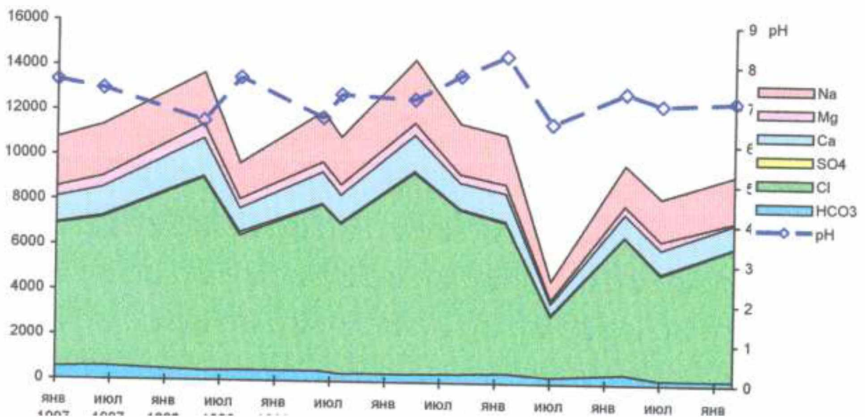
Рис.4.3 - Хімічний склад води в колодязі гр. Шугай (с. Качаново), мг/дм 3 (2019-2022 рр.)
