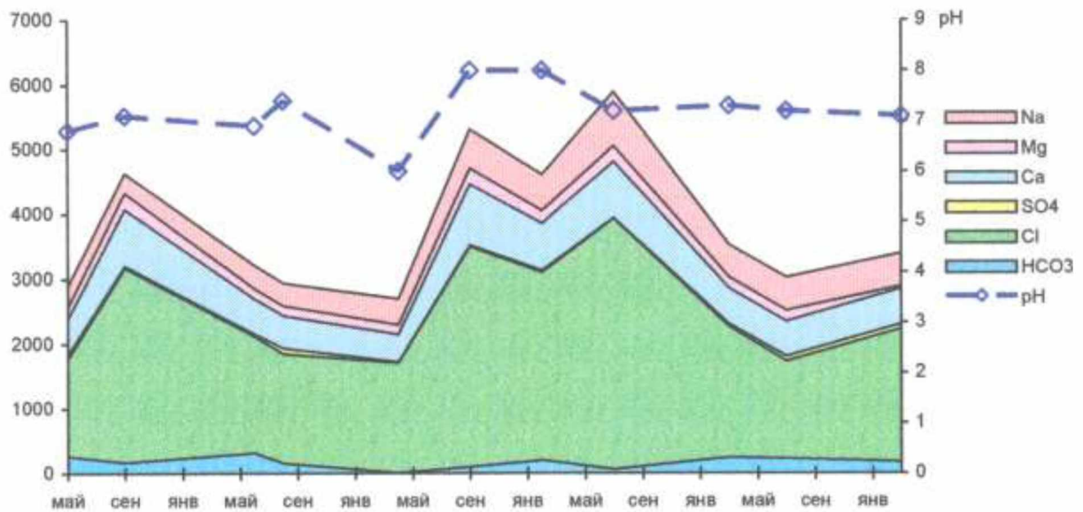
Рис.4.2 - Хімічний склад води в свердловині №29, мг/дм 3 (2019-2022 рр.)
