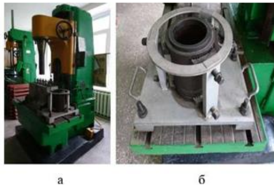
Рис. 2. Технологічне обладнання: а) вертикально-розточувальний верстат 2Е78П; б) пристосування для центрування гільз гідроциліндрів на станині верстату
