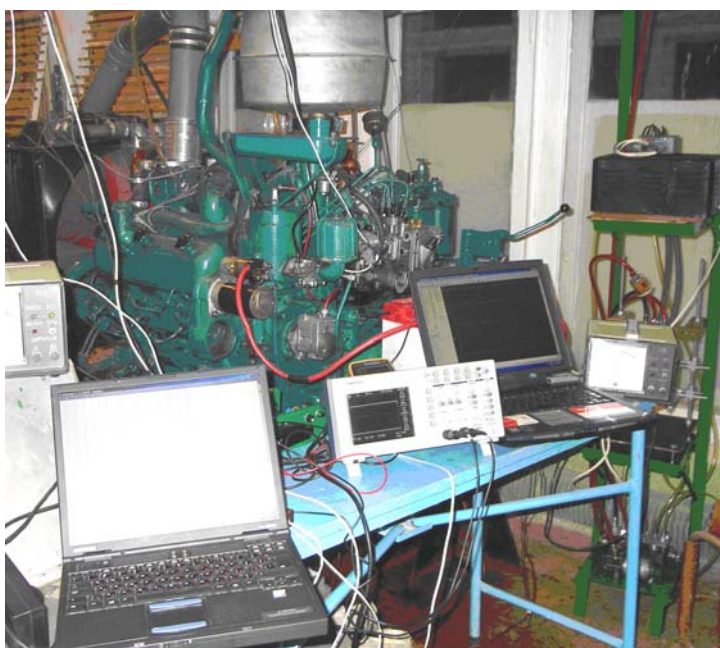
Експериментальні установки по дослідженню паливо-економічних і екологічних показників роботи автотракторних дизелів
