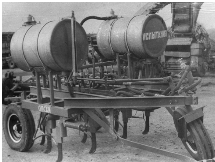
Пристрій для внесення РДК
