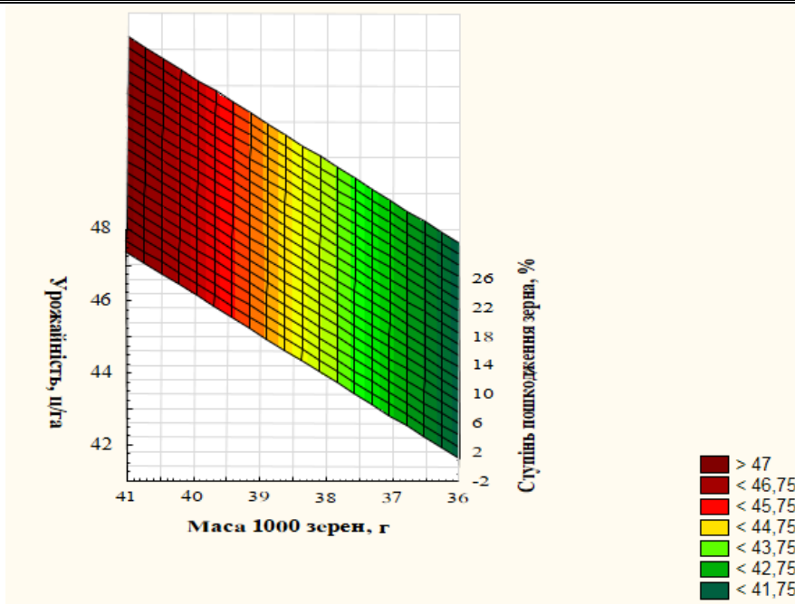
Рис. 1. Графік лінійної регресії урожайності пшениці озимої від ступеня пошкодження зерна та маси 1000 зерен
