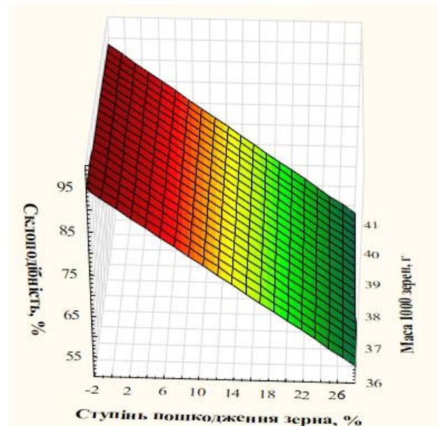
Рис. 3. Графік лінійної регресії склоподібності пшениці озимої від ступеня пошкодження зерна та маси 1000 зерен
