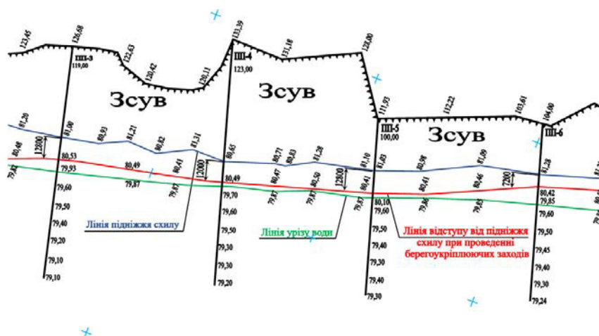
Рис. 2. Фрагмент схеми із створами ПП-3, ПП-4, ПП-5, ПП-6
