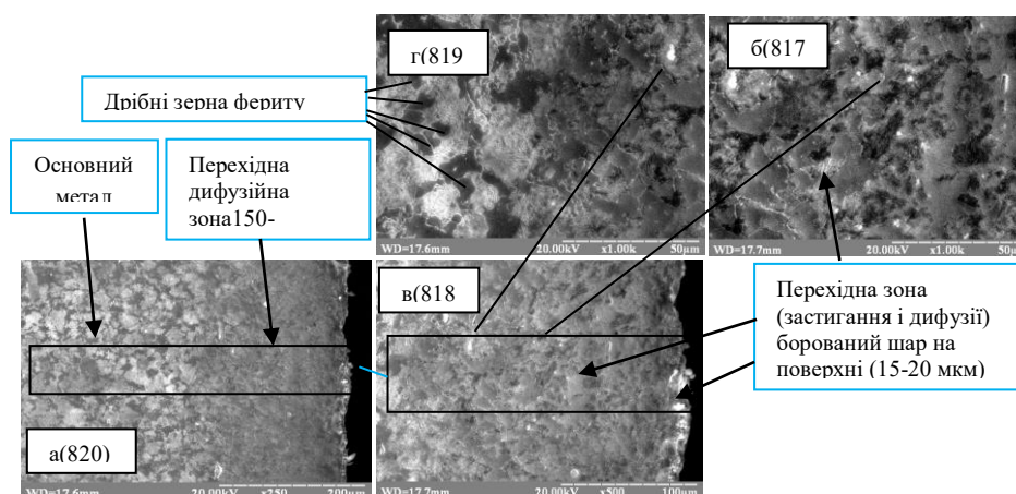
Рис.1. Фотографії мікроструктур сектора кулачка (а.(820), б.(819), в.(818) середини), б(813), г.(819) перехідної, підшарової і крайньої зони.
